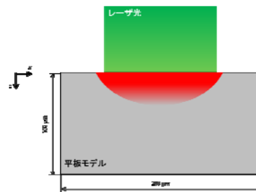
図4 熱伝導解析モデルの模式図
