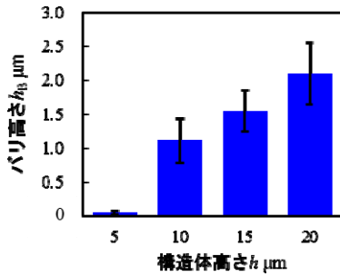
(a) 構造体のバリ高さの平均値 h_B
