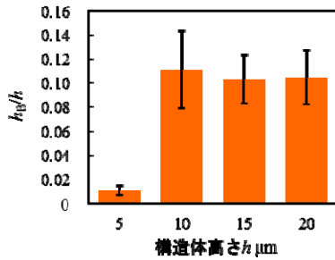
(b) h_B と構造体高さ h の比 h_B/h
