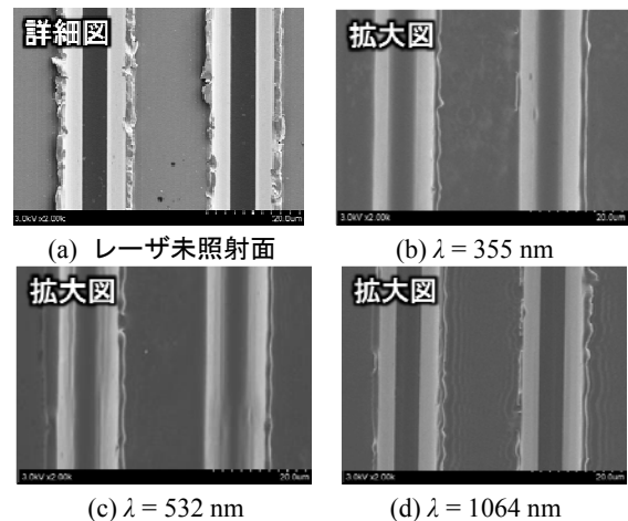
図 6 レーザー未照射面およびレーザー照射面の様子 (0.5 J/cm 2 , 200 shots)
