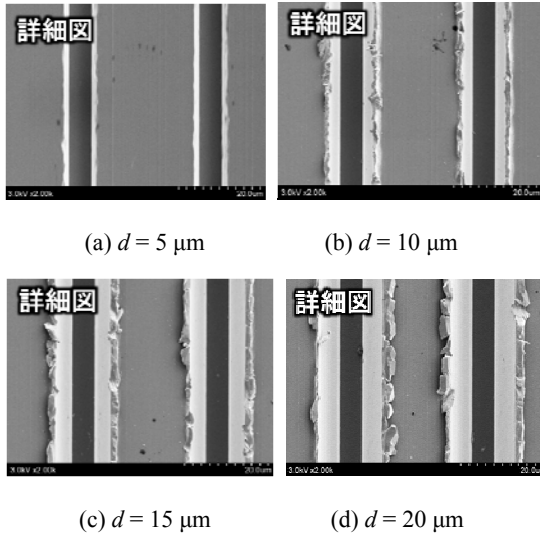
図2 矩形平行溝構造体に発生した欠陥の様子
