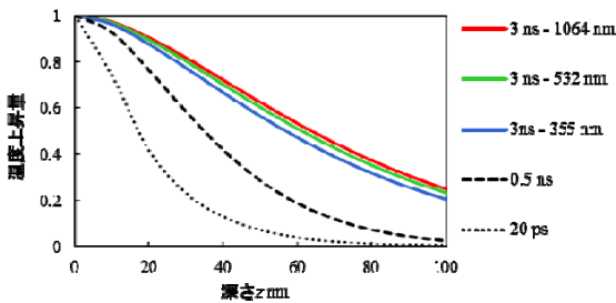
図 5 各条件でのレーザー照射による深さ方向の温度勾配
