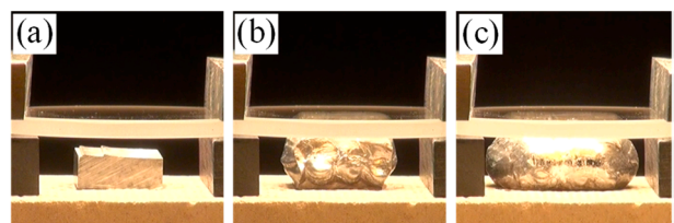
図3 光加熱によるプリカーサの発泡の様子。ガラス板を透過した光によりプリカーサを発泡。気孔を維持したままガラス板により上面への発泡を拘束している 25) 。
