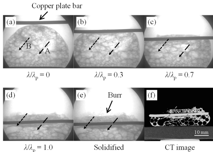
図 8 プリカーサ発泡直後のプレス加工を X 線透過により観察。(a)-(d)プレス加工中の様子。矢印で示した A, B の気孔は、位置は変わっているが、形状はほぼ維持されている。(e)凝固後の発泡アルミニウムの X 線透過画像と、(f)凝固後の発泡アルミニウムの X 線 CT 画像を比べると、X 線透過画像でも気孔を明瞭に観察できている。すなわち、発泡直後のプレス加工では気孔を維持しながら材料流動により発泡アルミニウムを形状付与できる 27) 。
