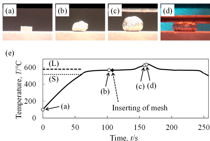
図5 プリカーサの発泡と発泡したプリカーサへのプレス加工の様子、およびその時の温度履歴。(a)-(c)母材の液相線温度を超えると大きく発泡する。(c)の上部に見えるものがプレス加工に用いたプレス金網で、加熱発泡中に導入している。(d)加熱終了直後に金網によりプレス加工することで形状付与でき、気孔が圧潰する様子も見られない。(e)液相線温度を超え大きく発泡し、発泡による膨張が止まったら、加熱をやめ((c)点)プレス加工を行う((d)点) 1) 。
