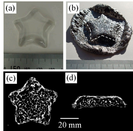
図 7 プレス加工による形状付与の一例。 (a)星形の型のモデル。(b)プレス加工により得られた星形状の発泡アルミニウム。(c)上方から観察した X 線 CT 画像。(d)横方向から観察した X 線 CT 画像。気孔が維持されている 23) 。
