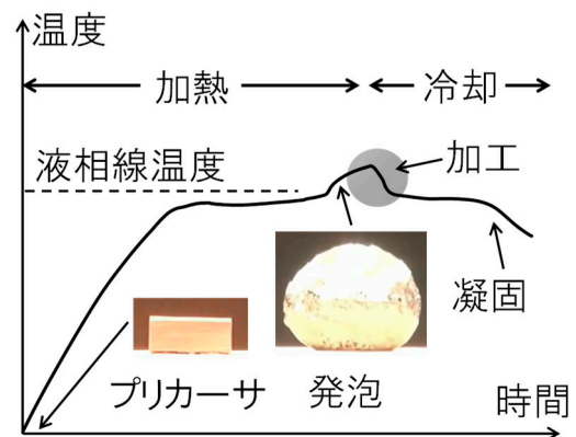
図2 プリカーサ法における発泡工程の温度履歴。灰色の部分为本稿で加工を試みた温度帯である。
