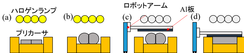
図 9 発泡直後のプレス加工による複数プリカーサの接合の概略図。(a), (b)2つのプリカーサをセラミックスの型に入れ加熱し発泡させる。(c), (d)加熱終了後、プレス金型であるアルミニウム板でプレス加工を行い接合する 24) 。
