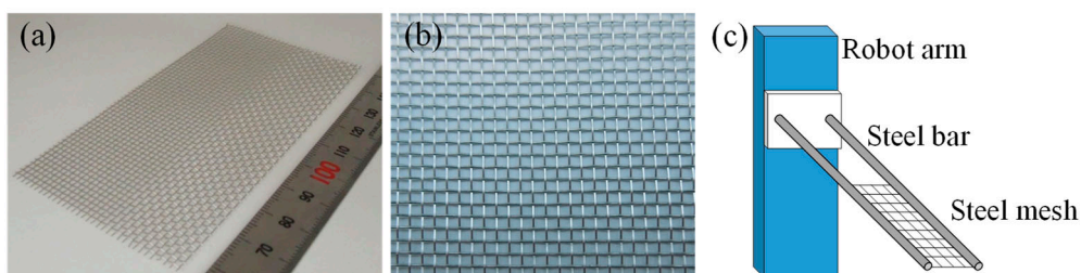
図4 (a)プレス金型に用いた金網。(b)金網の拡大写真。(c)金網をロボットアームに装着した概略図 1) 。
