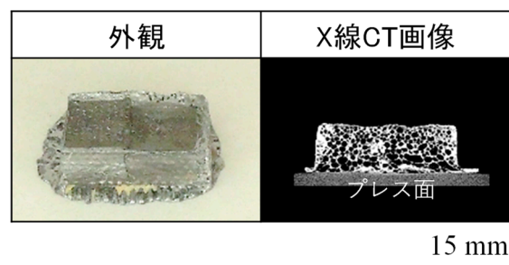
図 10 複数プリカーサの発泡直後のプレス加工により接合した発泡アルミニウムの外観写真と X 線 CT 画像。外観写真の表面には若干の接合線が見られるが、X 線 CT 画像から内部には接合線が見られず気孔も壊れることなく維持されている 24) 。
