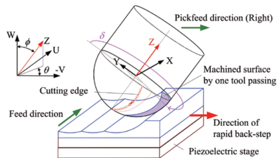
図1 実験装置の位置関係と座標軸の定義
