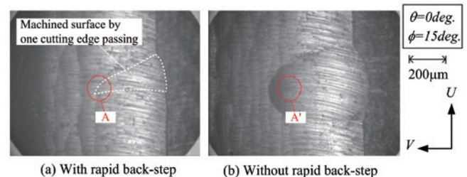
図4 急速後退によって観察される工具刃先通過痕形状
