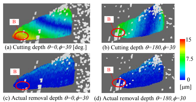
図7 工具切れ刃通過時における工具切込深さと実際の除去深さの相違 ( \theta = 0 度および 180 度の場合)
