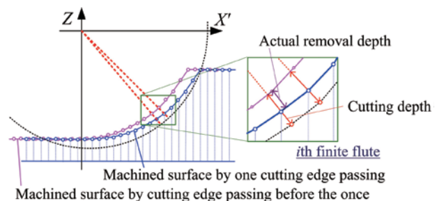
図2 工具切れ刃通過位置の比較による除去深さ推定
