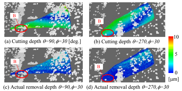
図6 工具切れ刃通過時における工具切込深さと実際の除去深さの相違 ( \theta = 90 度および 270 度の場合)
