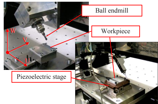
図3 実験機器の構成
