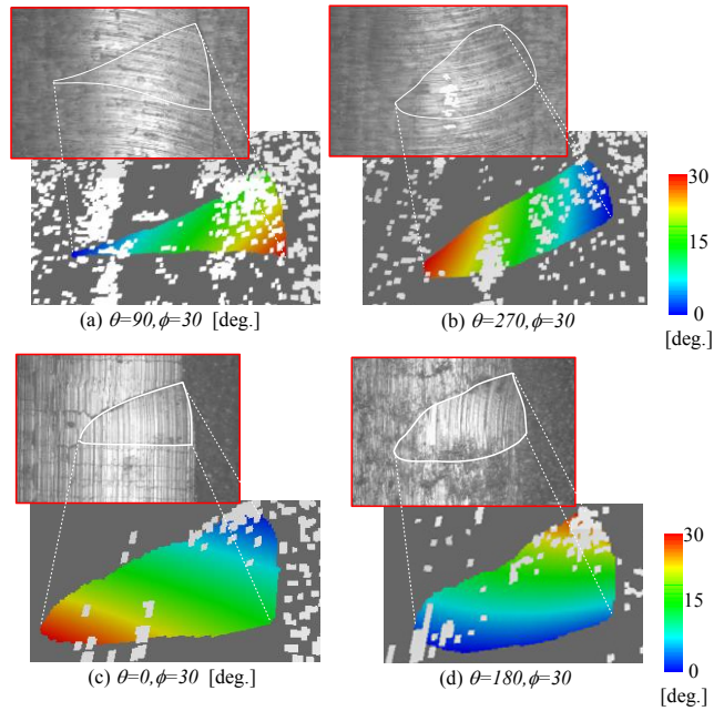
図5 工具姿勢における工具切れ刃通過方向の変化
