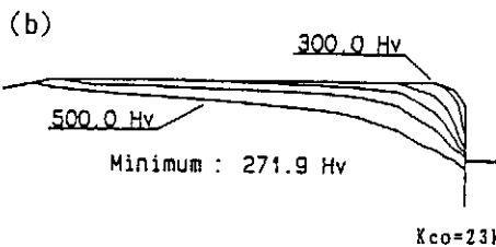
図8 下型インナー表面近傍の (a) 温度分布、 (b) 2500回鍛造後の熱軟化（硬さ分布） の評価結果（有限要素解析）
