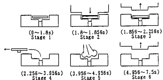
図2 鍛造1サイクル中のプロセスの連鎖
