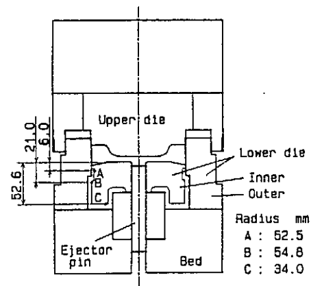
図1 閉塞鍛造模型と熱電対温度計測位置
