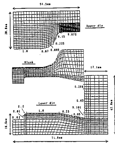
図6 非定常温度場の解析に用いられた有限要素分割例(数値は接触時間割合)
