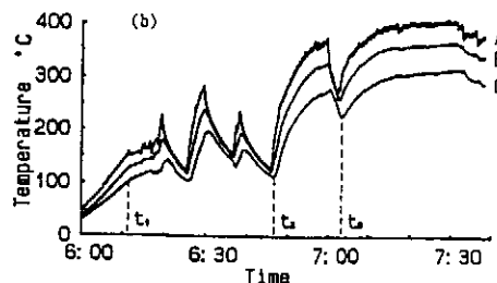
図3 (a) 鍛造1サイクルに計測点A(図1)で計測された温度(定常熱サイクル) (b) 計測点A,B,Cで計測された温度履歴
