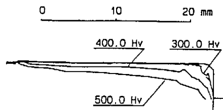
図10 2500個鍛造後の下型インナー表面近傍の実測硬さ分布
