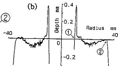
図4 鍛造数2500で、(a)図1の下型インナー鍛造型表面近傍に発生したヒートクラック(斜め切断角7度) (b)下型インナー鍛造型表面の摩耗プロフィール
