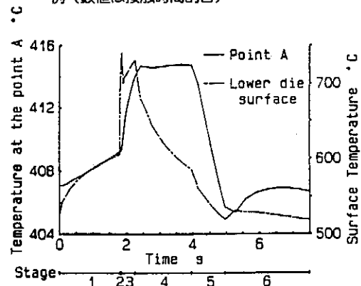
図7 下型インナー点Aおよび下型丸み部入口表面の熱サイクル評価結果(有限要素解析)
