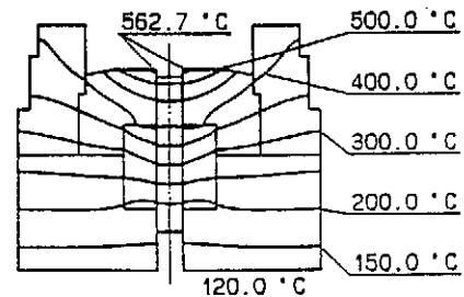
図5 下型の準定常温度分布計算例(図3の時刻7:25にほぼ対応)
