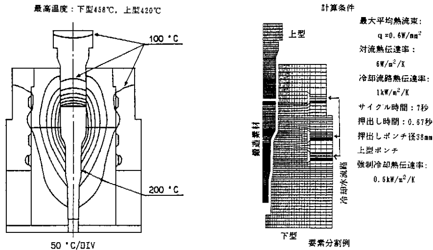
図 11 前方押し温度制御(寿命評価)用鍛造型の略図と定常温度場の評価例：ポンチおよびダイスの冷却が特に重要となる。表面からの冷却時間の確保、ダイス内部からの冷却、プレスダイセットからの冷却が制御のために必要になる。
