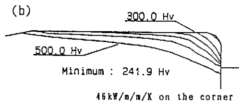
図9 下型インナー表面近傍の (a) 温度分布、 (b) 2500回鍛造後の熱軟化（硬さ分布） の評価結果：図8でコーナー部の接触熱 コンダクタンスを2倍に評価した場合
