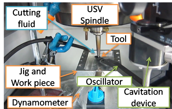
図4 複合超音波加工の実験装置図
