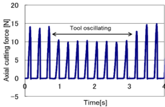
図1 超音波振動の援用によるスラスト力の低減
