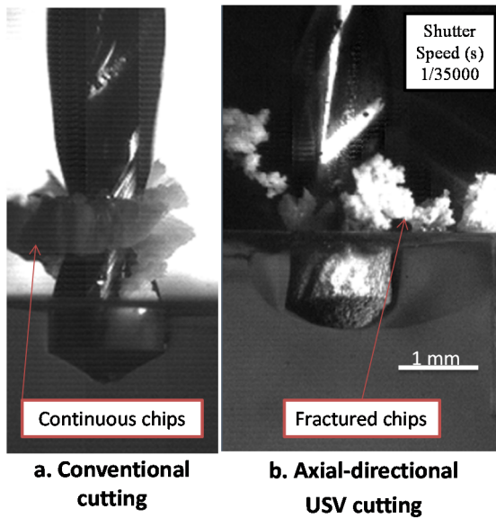
図5 慣用加工と超音波振動切削における切りくず生成の比較
