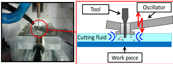
図2 キャビテーション援用加工
