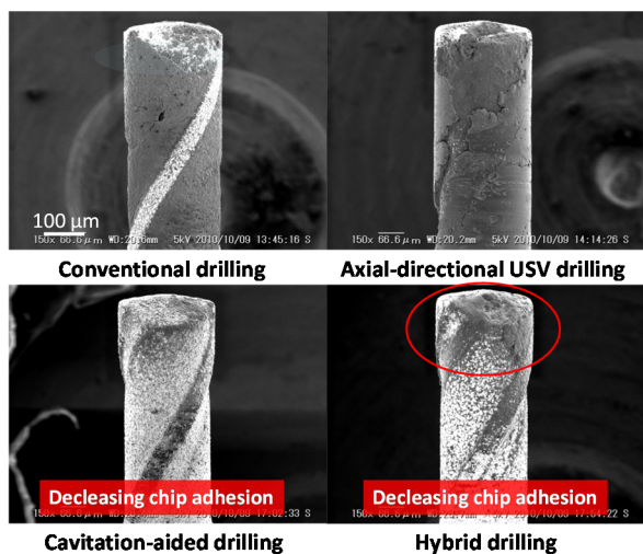
図8 工具側面の観察結果（10穴加工後）
