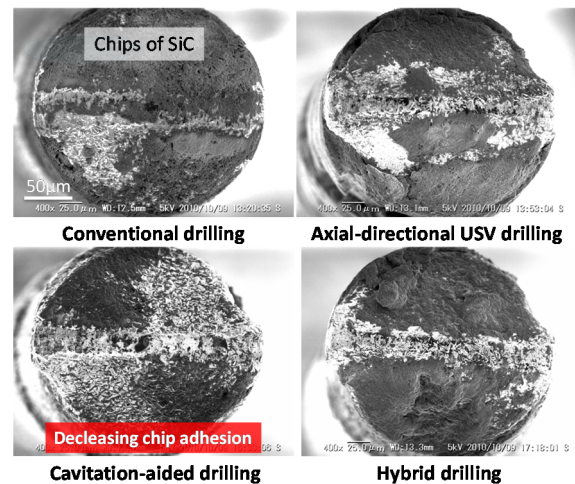
図7 工具底面の観察結果(10穴加工後)
