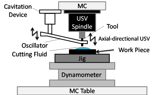
図3 実験装置のモデル図
