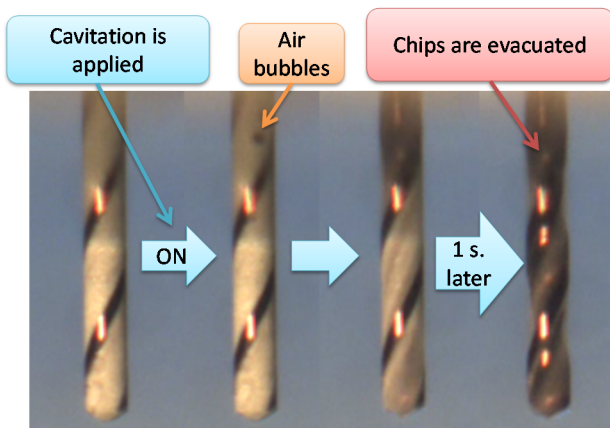
図6 キャビテーション発生時の切りくず排出性
