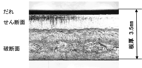
図8 マイクロスコープによる分離面観察例
