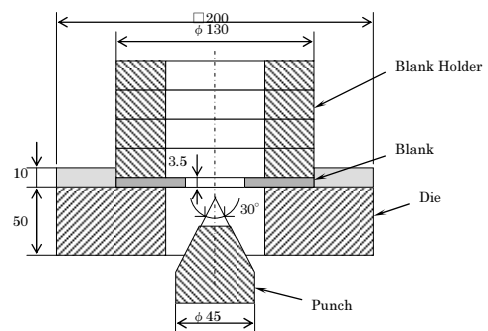
図 4 穴広げ実験工具の組立図
