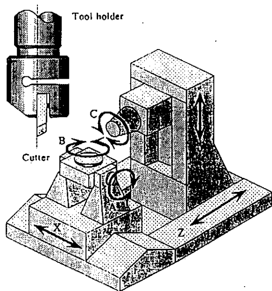
図2 6軸制御マシニングセンタ
