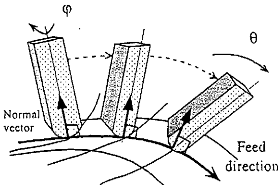
図11 工具姿勢の連続変化の概念図
