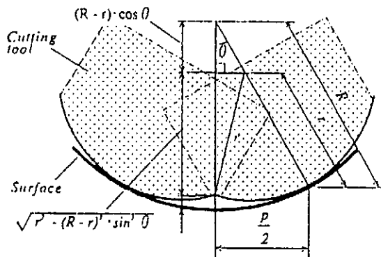
図4 カスプ高さの計算
