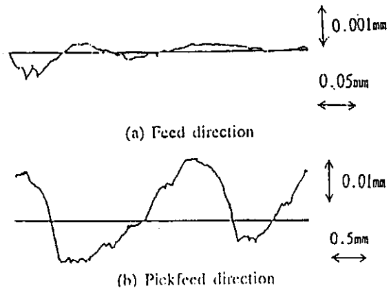
図17 表面粗さの測定結果
