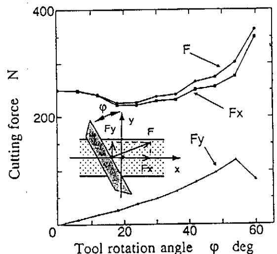
図12 角度 \phi と切削力 F の関係
