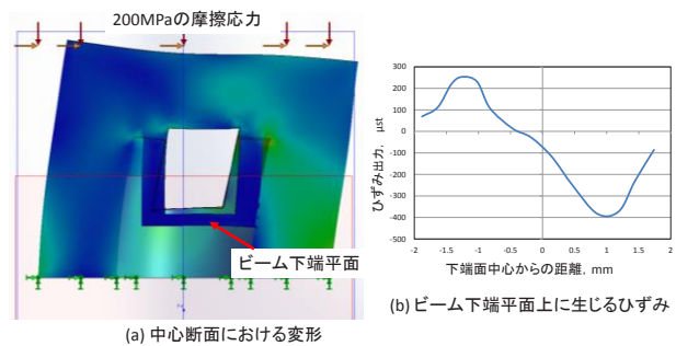
図4 摩擦センサへの摩擦応力負荷に対する変形とひずみ出力の解析例
