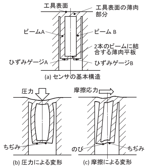
図 1 摩擦センサの基本構造と検出原理
