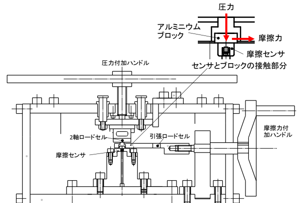
図7 摩擦センサ出力の検定装置
