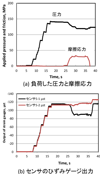
図8 圧力・摩擦センサの検定出力例
