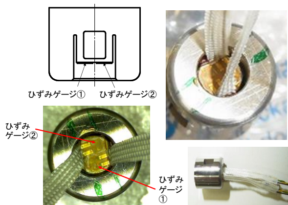
図6 圧力・摩擦センサブロックへのひずみゲージ貼付け
