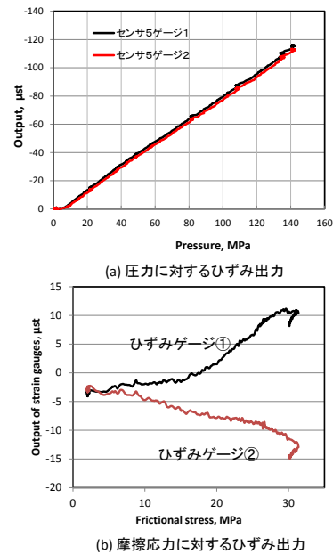
図9 圧力および摩擦応力に対するひずみ出力の例
