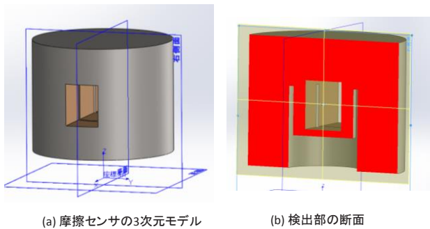
図2 摩擦センサの3次元モデル
